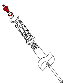
Kit 1: Bremsnockenwellen-Kit mit Exzentermutter ersetzt durch Kit 2
