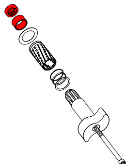
Kit 2: Bremsnockenwellen-Kit mit Exzentermutter und Distanzhülse ersetzt Kit 1
