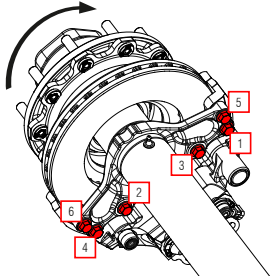
Ohne Passschraube
