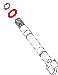
Version mit Sicherungsring und Scheibe
