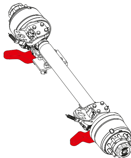
Zwangsgelenkte Achsen (ZL) mit Lenkhebel für hydraulische oder mechanische Lenkung
