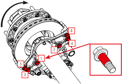
Mit Passschraube
