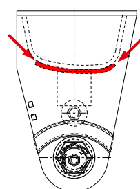
Vordere Aufhängung
