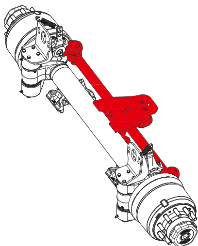
Nachlaufkachsachsen (NL) mit Spurstange, Stabilisierungs- und Verriegelungseinheit
