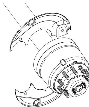
Geschraubte Version mit Sicherungsmutter / Schraube und Scheibe
