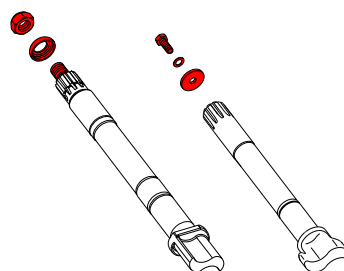
Geschraubte Version mit Sicherungsmutter / Schraube und Scheibe
