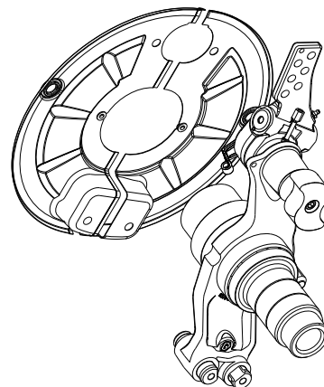
Geschraubte Version durch Bremsenträger (GEOKH2)
