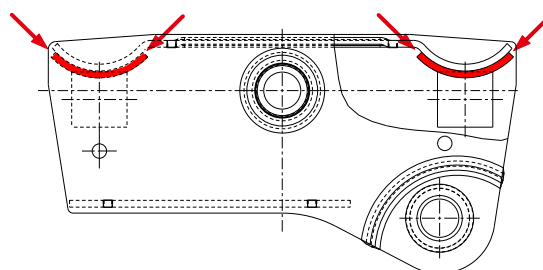
Ausgleichswiege
