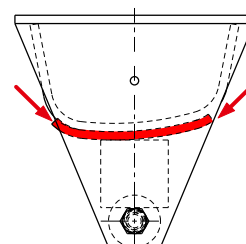
Gleitschuh
