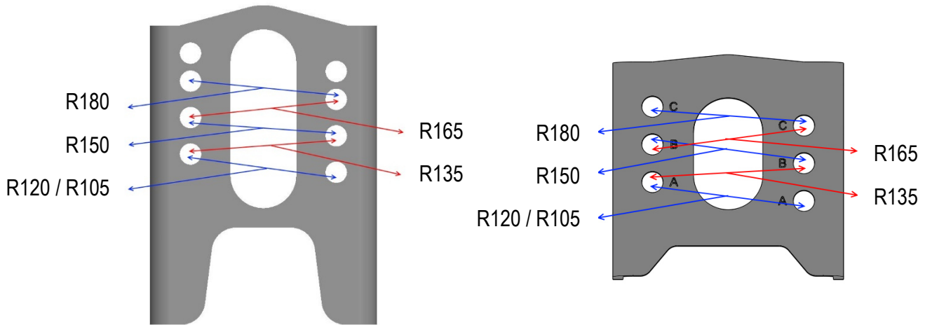
Beispiele Starrachsen: Lochbilder der Grundplatten
